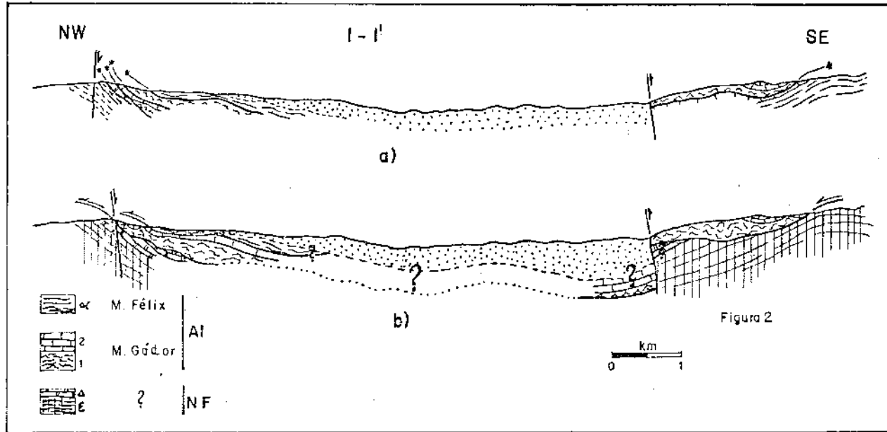
Fig. 2. a) Corte I-I' de la hoja de Tabernas.
