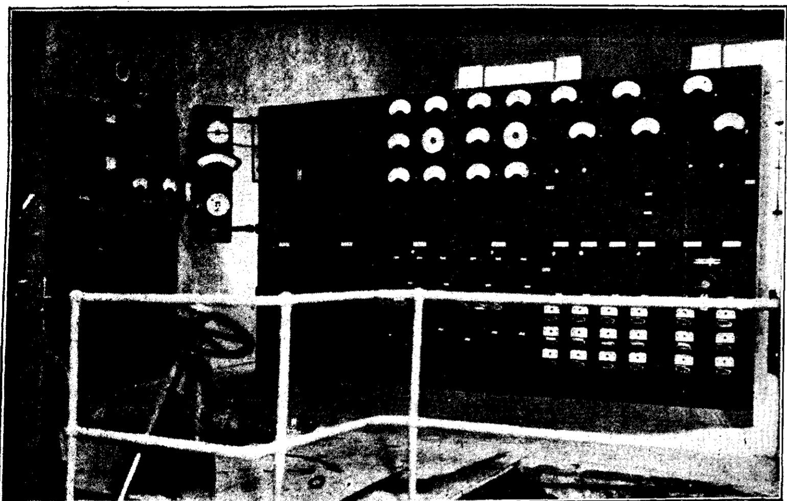
Cuadro de maniobras, de la central de Vélez
