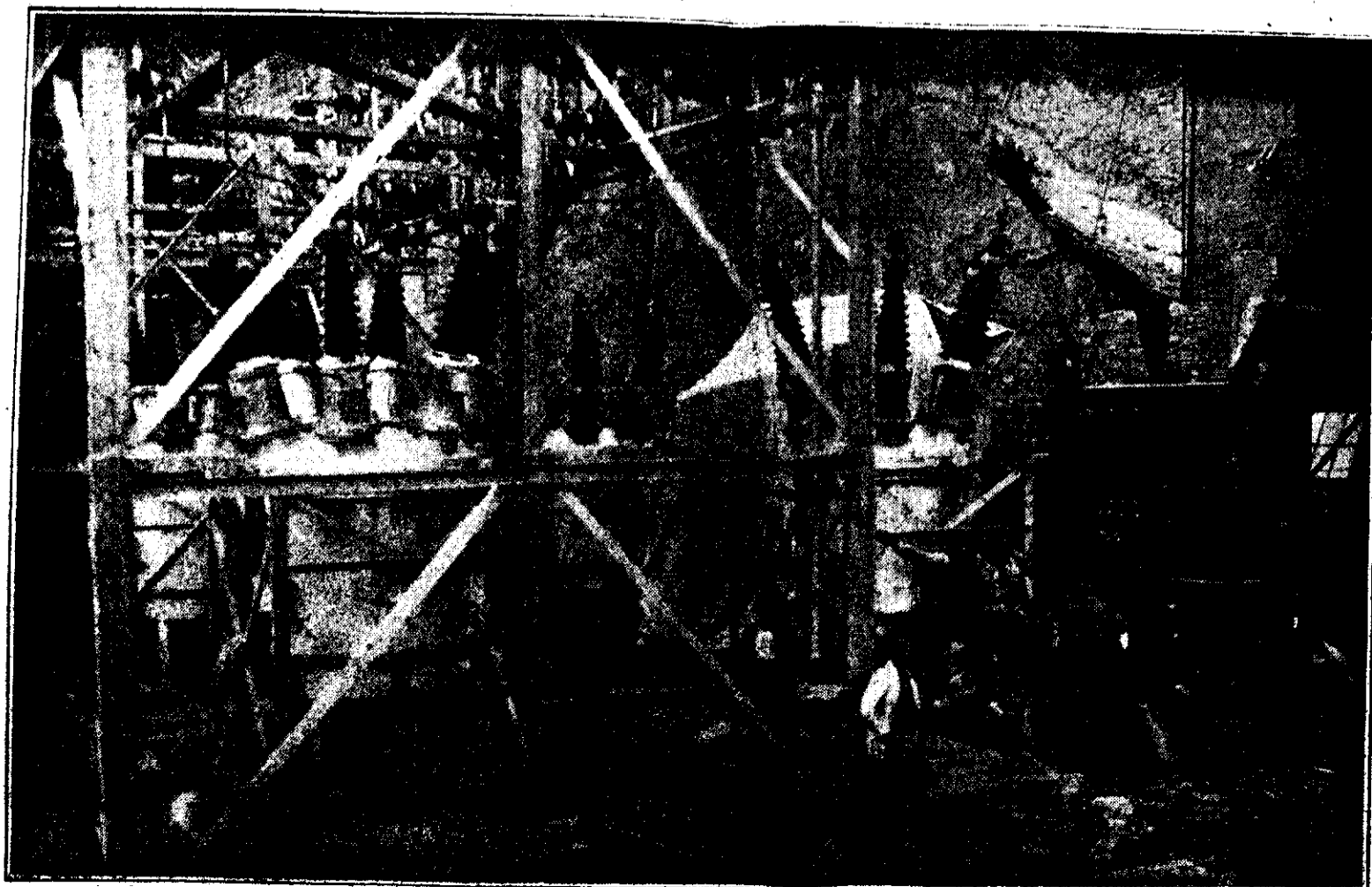
Instalación a la intemperie de interruptores automáticos en aceite y transformadores de circulación de aceite, forzada.
