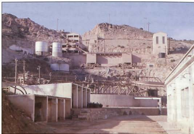
Figura 10. Planta Denver en funcionamiento en el año 1964 (gentileza de Antonio Arribas Moreno)
