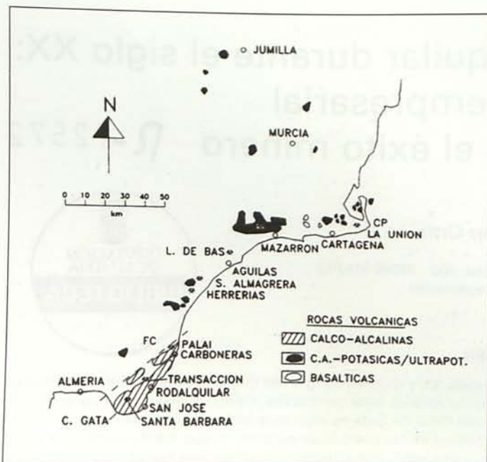
Figura 1. Situación geográfica y geológica de Rodalquilar (Castroviejo, R. 1998) Figure 1. Geographical and geological location of Rodalquilar (Castroviejo, R. 1998)
