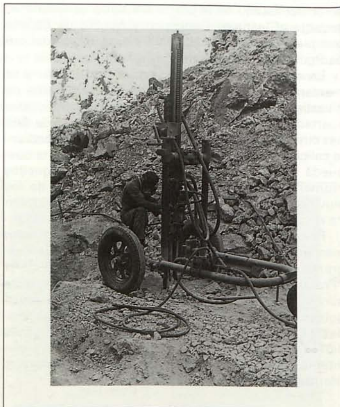
Figura 8. Wagondrill trabajando en las minas a cielo abierto del Cerro del Cinto en el año 1956 (Archivo de Escuela de Ingenieros de Minas de Madrid)
