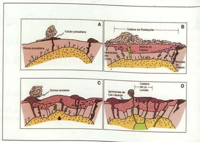
Figura 2. Formación del complejo de calderas de Rodalquilar (Arribas Rosado, A. 1993) Figure 2. Generation of the Rodalquilar caldera complex (Arribas Rosado, A. 1993)
