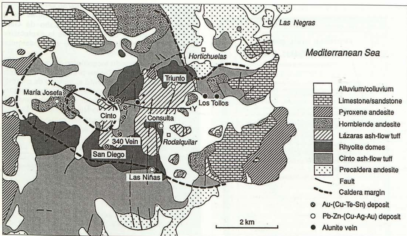
Figura 3. Situación de las principales minas de Rodalquilar y su relación con la geología del complejo de calderas (Arribas Rosado, A. 1995)
