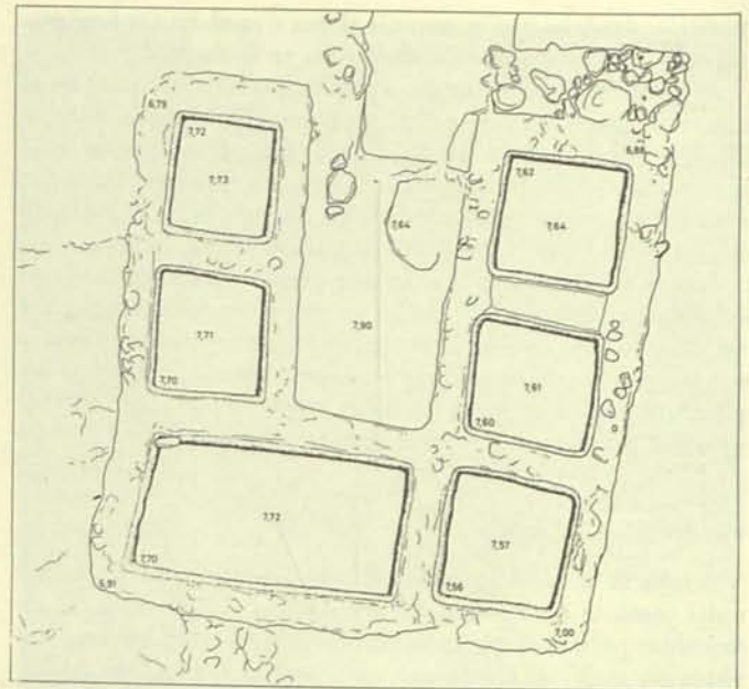
FIG. 2. Planta Balsas de Salazón. Corte I.
