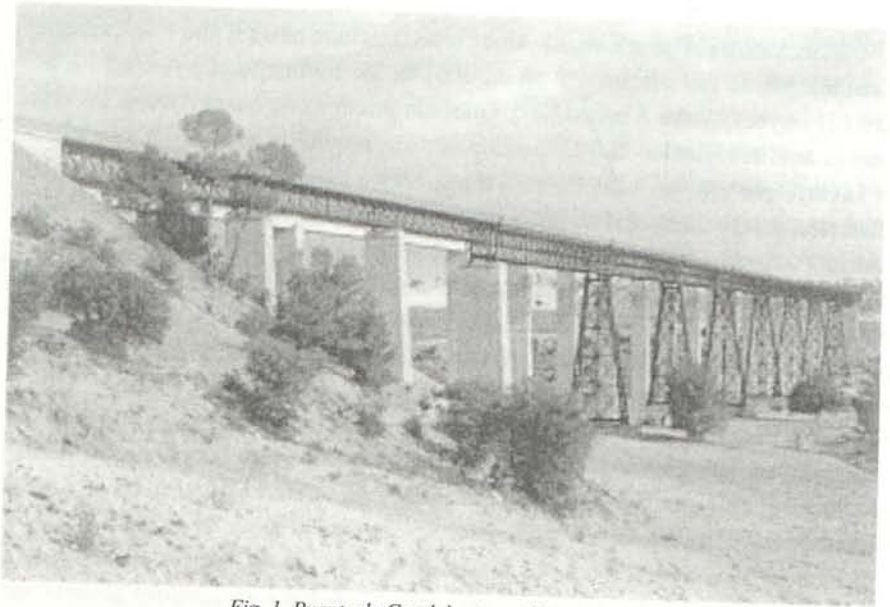
Fig. 1. Puente de Guadahortuna. Vista general.
