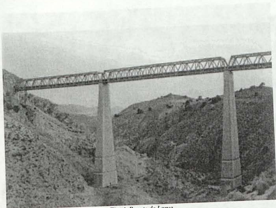
Fig. 4. Puente de Larva.
