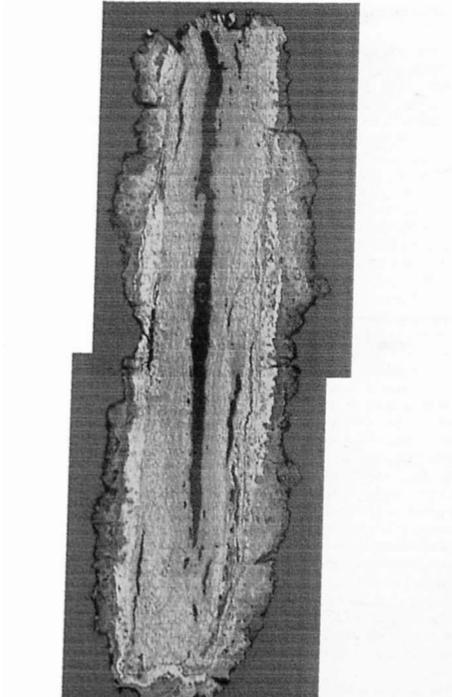
Fig- —LM-6146S (Pp. 122X) Huellas de forja laminares con la típica formación de huecos en el centro junto a la corrosión. Se ha consenado muy poco melal. Los productos de oxidación (sobretudo cuprita y "magnetita" consena de forma residual las estructuras originarías del metal. Ancho de la toma de aproximadamente 5 mm
