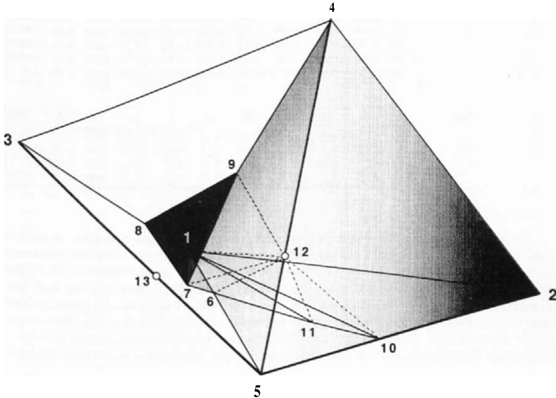
Fig. 4.—Tetraedro doble Cu-As-O-S/Cu-Fe-O-S (porcentaje molecular).
