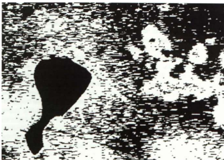
F.g 3 - a) LM-61025 <Pp 1287 , Inclusiones redondeadas de fases oxidantes en cobre metil.co Fotografía en B/N de una toma en color de luz reflejada digital.zada. b) LM-61287 (Pp 1287 , Separación cromática azul rojo del original en rojo de la Fig. 3a. Rojo= coloreado en rojo. Blanco= coloreado en azul Tanto el cobre de la masa básica como las inclusiones de las zonas que se han podido aislar muestran claras diferencias de color El cobre de color rojizo pobre en arsénico contiene cuprita de color azul En el cobre neo en arsénico de color azul existen inclusiones de "una fase de Cu_2O \cdot As_2O_3 " de color rojo
