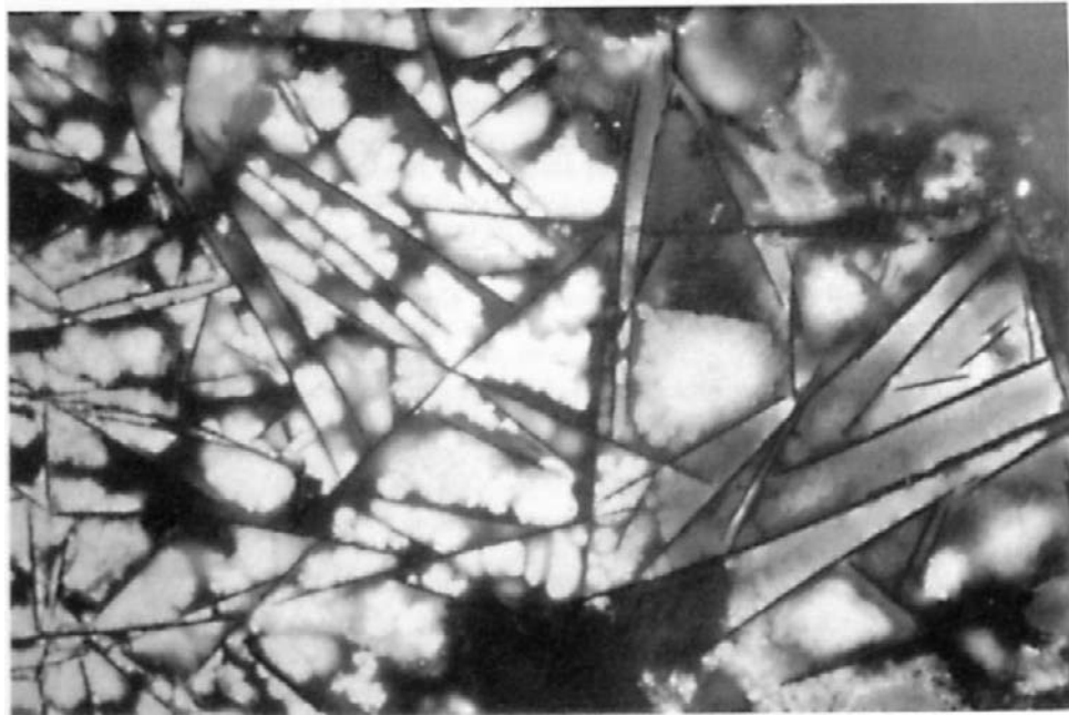
Lám. I.—a) LM-89342 (Pp. 1158) , toma n.º 2368. Fragmento cerámico en contacto con escoria fundida. La cerámica contiene silicatos ricos en Fe en diferentes estadios de transformación. Margen izquierdo: marrón oxidado o incoloro. Margen derecho: fundiéndose bajo una formación de burbujas. Luz reflejada, campo oscuro sin polarización. Ancho de la toma de aproximación 0.7 mm b) LM-89342 (Pp. 1158) , toma n.º 2369. Silicato laminar rico en hierro en fase de fundición. En contacto con las escorias de fundición se forman cuerdas orientadas de magnetita. Luz reflejada I polarización. Ancho de la toma de aproximadamente 0.28 mm
