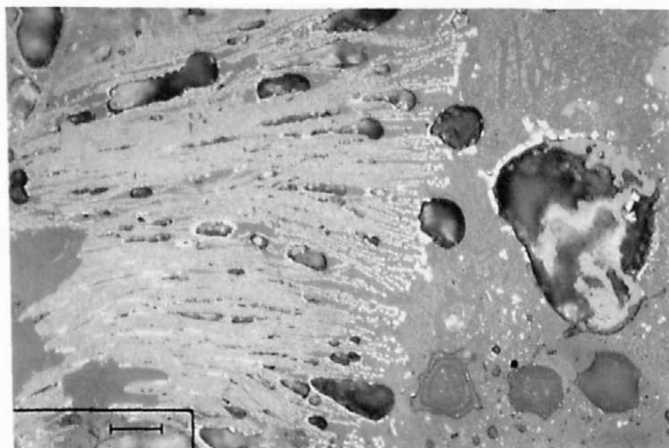
Lám. II.—a) LM-76083 ( Pp. 1154 ). toma n.º 2362. Escoria de fundición formada in situ en el fragmento cerámico, con inclusiones de numerosas gotitas de hierro. Luz reflejada, sin polarización. Ancho de la toma de aproximadamente 2.8 mm. b) LM-89407 ( Pp. 1155 ), toma n.º 2149. Varillas de delafosita ( \text{CuFeO}_2 ) en una matriz vidriosa. El vidrio de la escoria contiene gotitas muy pequeñas de cobre (de color amarillo) en forma dispersa. Luz reflejada, campo oscuro sin polarización. Ancho de la toma de aproximación 0.28 mm.
