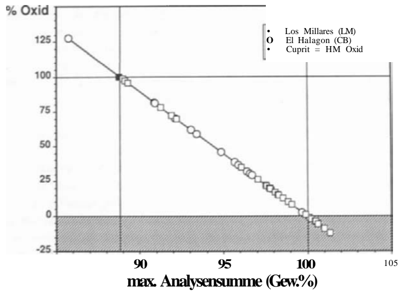
Fig. 5.—Suma de los análisis metálicos de LM y CB (valores máximos) según referencia de Hook et al. (1991) (Tablas 1 y 2). El grado de descomposición derivado sobre la base de Cu_2O=100\% .
