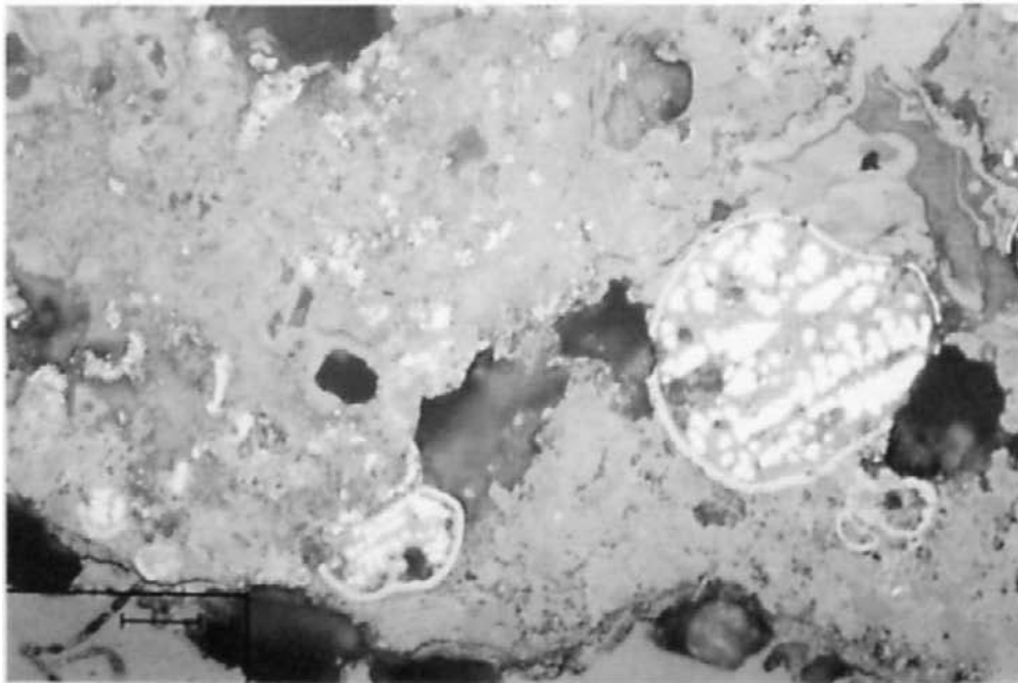
Lám. 111.—a) LMS9381 ( Pp. 1160 ). toma a' 2382. Se aprecia el contacto entre la cerámica y la escoria de fundición. En la cerámica se funde un paquete de silicatos laminares. Se forma una fundición nca en SiG*, que al enfriarse se transforma en vidrio con inclusiones de piroxeno (de color verdoso). El vidrio de la escoria contiene nubes de gotitas metálicas muy finas de cobre de color amarro-rojizo. Luz reflejada, campo oscuro sin polarización. Ancho de la toma de aproximadamente 0.7 mm. b) LM-33119 ( Pp. 1219 ). Bolita de escona rica en magnetita y metal descompuesto prácticamente en su totalidad. Ambas panes están adheridas. La bolita -metálica" es muy porosa y contiene en la cubierta de escona originaria aún algunos sulfure» de Cu-Fe-Zn. Ancho de la toma de aproximadamente 4.5 mm.
