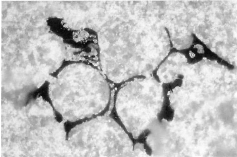
Lám. V.—a) LM-61025 ( Pp. 1287 ). toma n.º 2146. Cobre metálico en proceso de oxidación. En la transformación del cobre a \text{Cu}_2\text{O} se libera plata metálica en forma de partículas muy finas de color blanco. Luz reflejada. I polarización. Ancho de la toma de aproximadamente 0.7 mm. b) LM-33III8 ( Pp. 1282 ). toma n.º 2186. Cobre metálico con masa intergranular eutéctica. El cobre metálico y las líneas que recorren la masa intergranular están totalmente descompuestos. Luz reflejada en lubricante. I polarización. Ancho de la toma de aproximadamente 0.14 mm.
