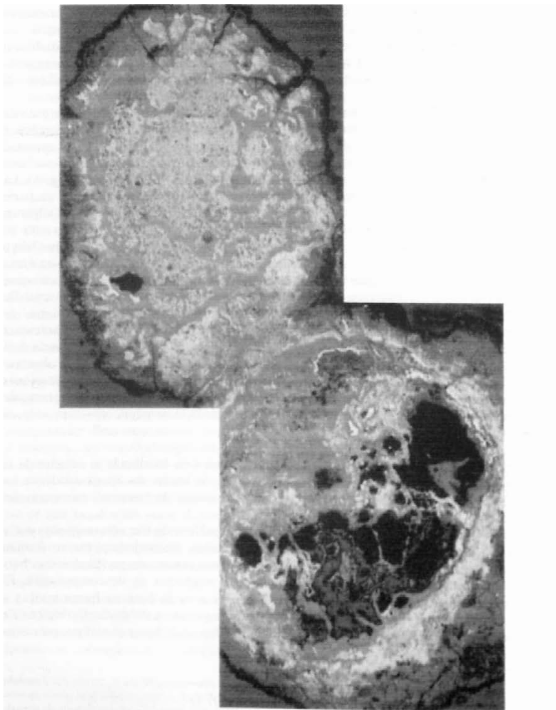
Fig. 1.—CB-683 (Pp. 1147), toma n.º 2311. En la escoria existen inclusiones de mineral de sulfuro de cobre. En las fisuras se aprecia digenita/calcosina en el inicio de su transformación a covellina. Luz reflejada. I polarización. Ancho de la toma de aproximadamente 0,28 mm.
