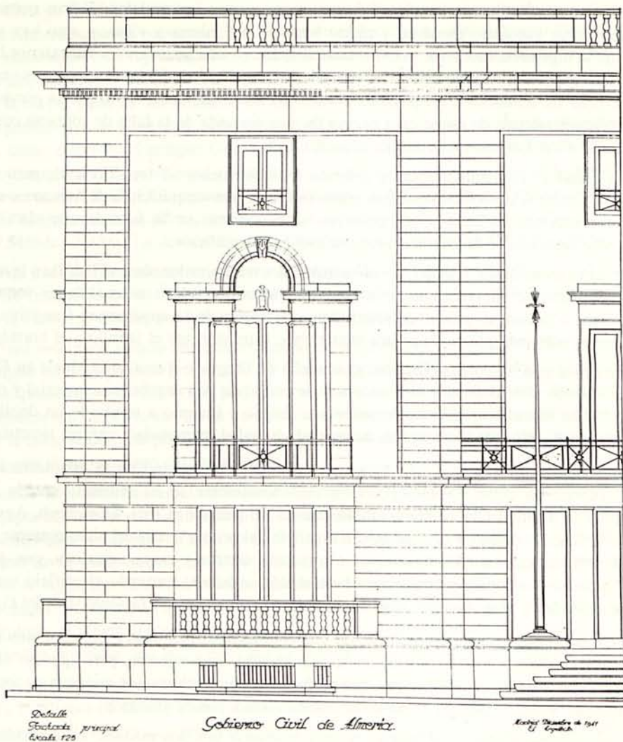
Fig. 6.- Detalle de la fachada principal
