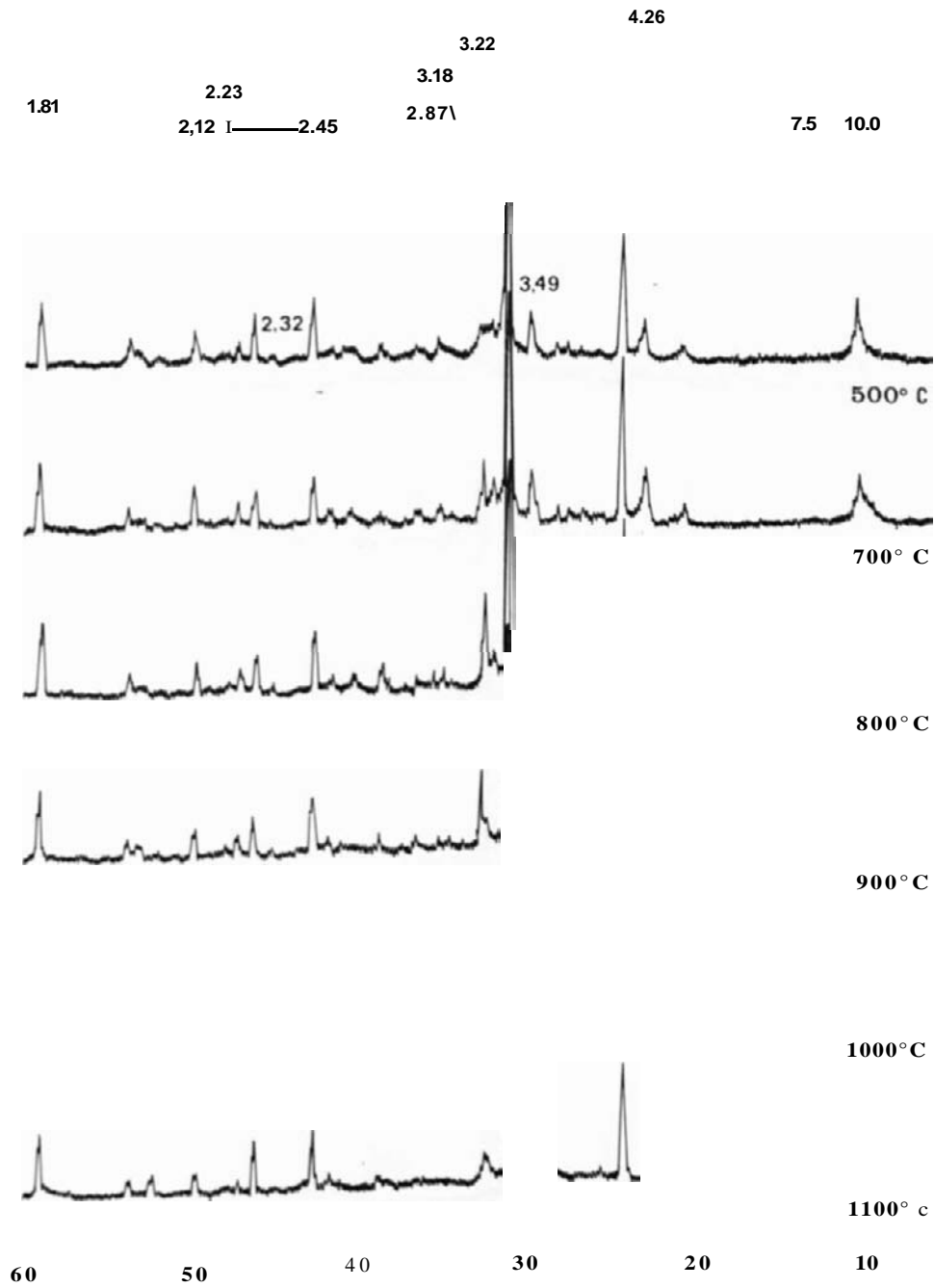
Fig. 7—Pieza n.º 2. Diagrama de difracción de rayos X. Método de Debye-Scherrer.
