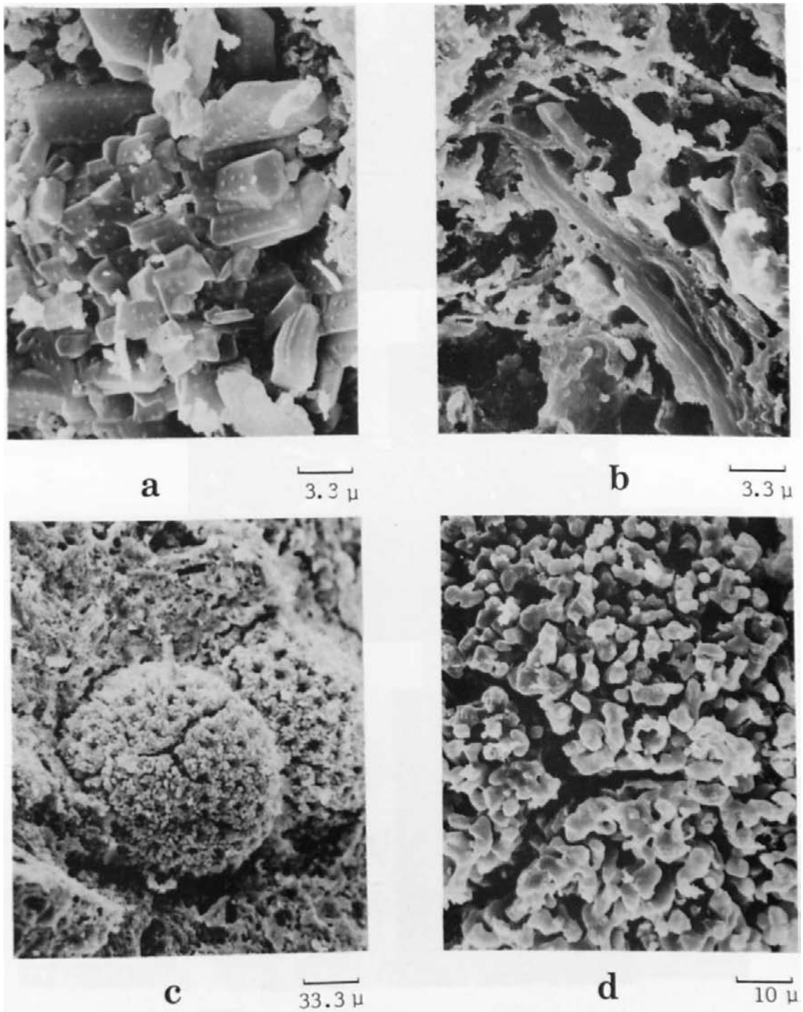
Lám. IV.—MEB. Pieza n.º 28. Zona externa, cristales con Potasio y Calcio (a). Zona interna, detalle (b). Zona externa, glóbulos de \text{CO}_3\text{Ca} (c). Zona externa, detalle de los glóbulos de carbonato (d).
