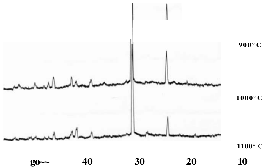
Fig. 9—Pieza n.º 14. Diagrama de difracción de rayos X. Método de Debye-Scherrer
