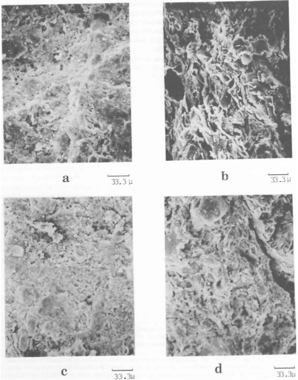
Lim I - MEB Pieza n* 2. zona externa (a) e interna (b) Pieza n.* 18. zona externa negra (c) e interna (d).
