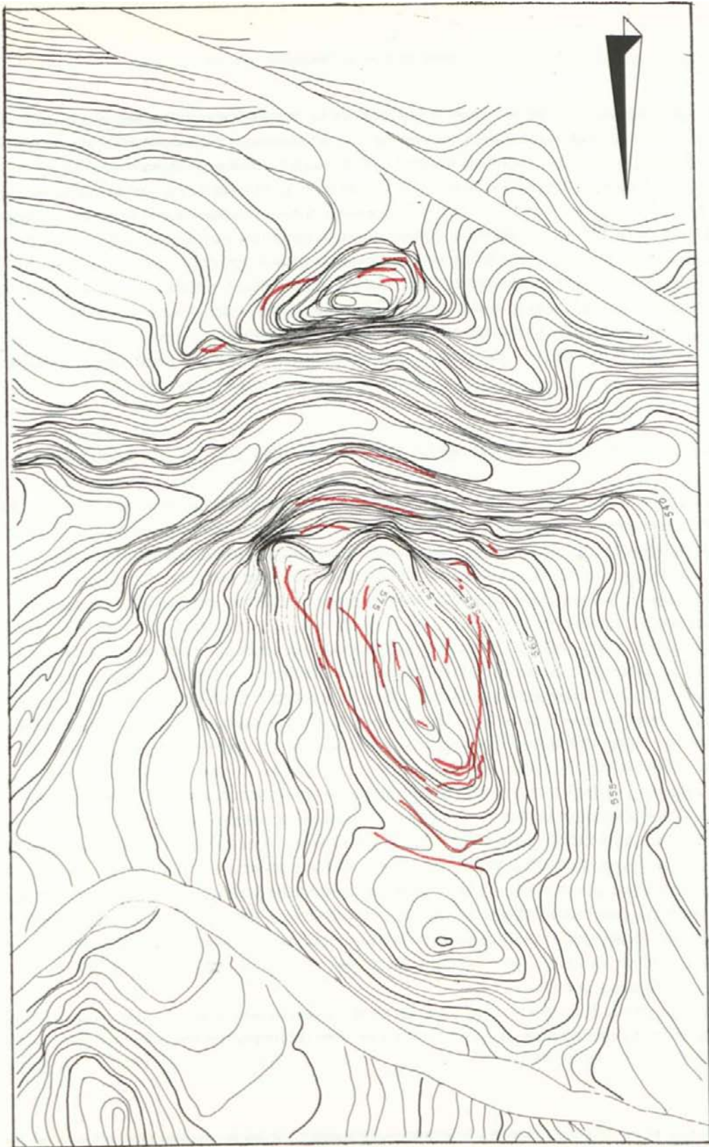
Fig. 4.—Levantamiento topográfico del Cerro del Nacimiento con la localización de las estructuras (en rojo).
