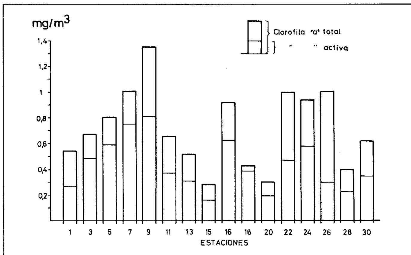
Figura 12.— Concentración de clorofila total y activa, en algunas estaciones litorales, durante la campaña de Agosto.
