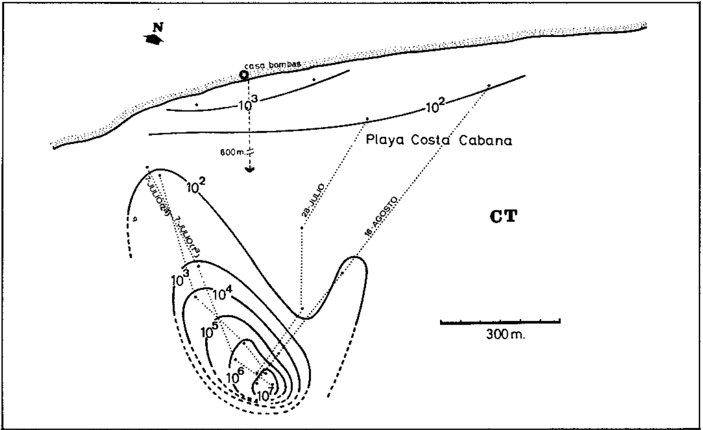
Figura 4.— Patrones direccionales de dispersión en cada una de las campañas realizadas (.....), e isolneas de concentración de coliformes totales.
