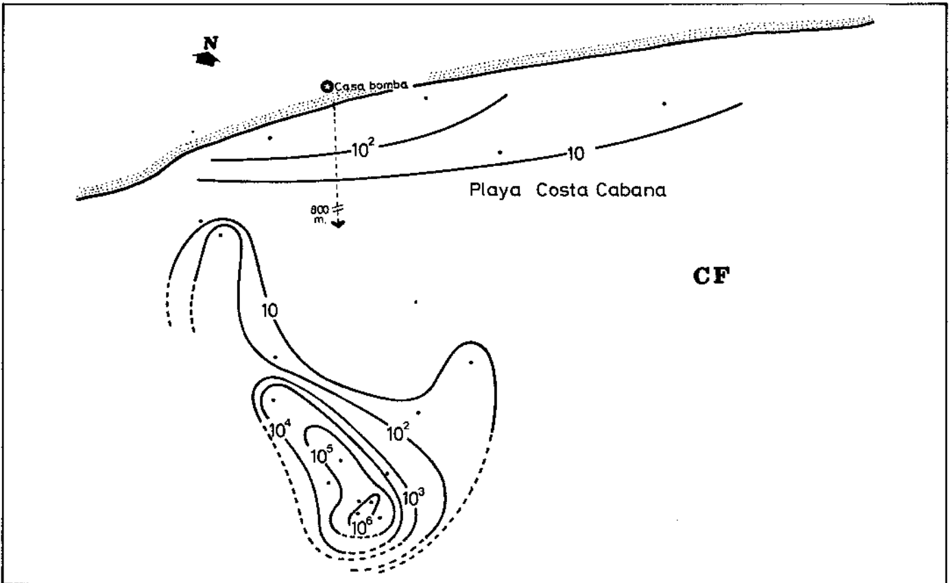
Figura 5.— Isolneas de concentración de coliformes fecales.
