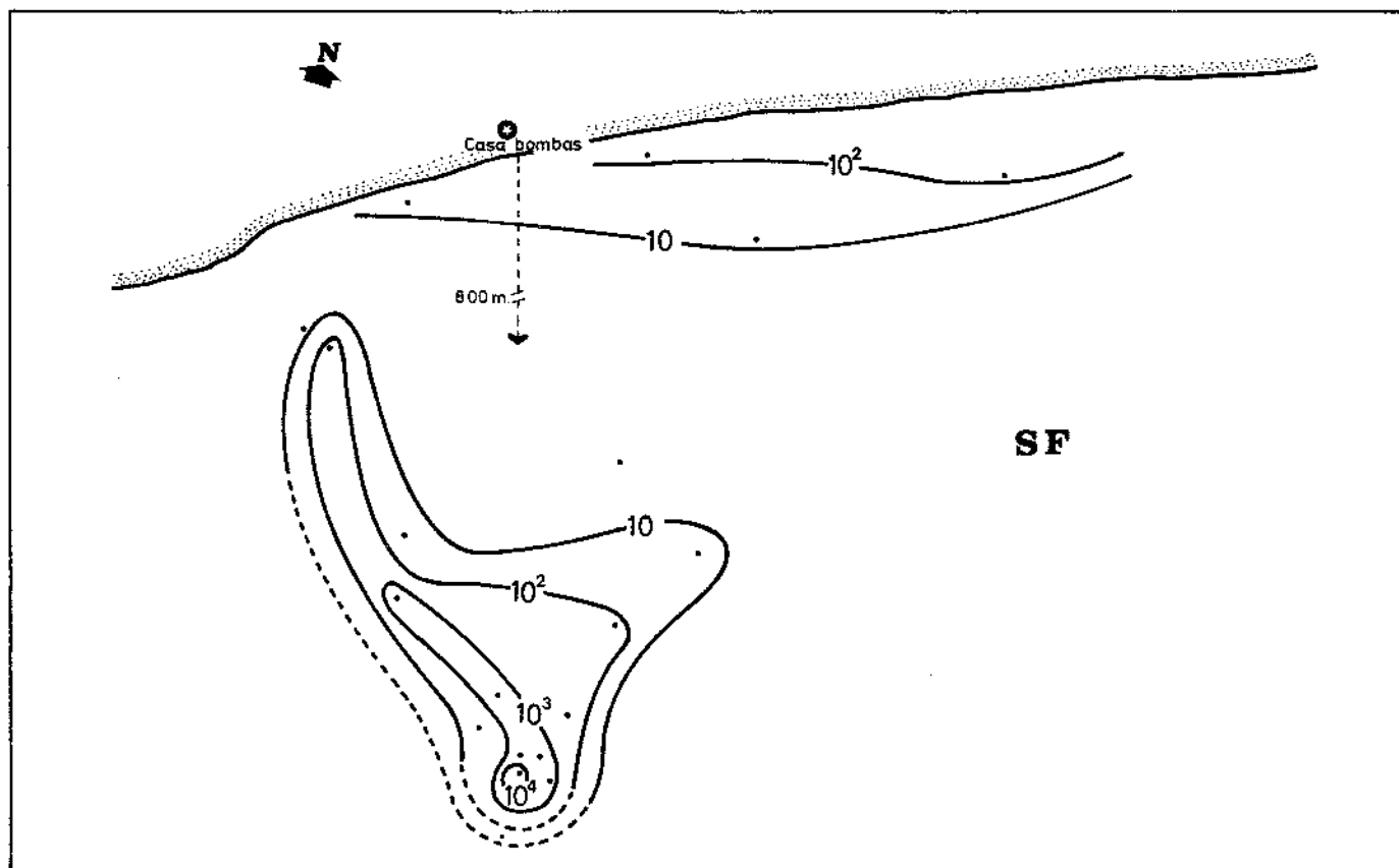
Figura 6.— Isolneas de concentración de streptococos fecales.
